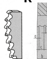
Esecuzione rompitruciolo
