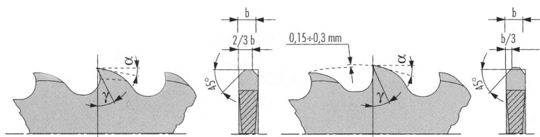
Esecuzione standard
